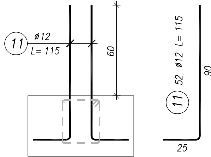
K-1 wykotwienie rdzeni skala 1:25
