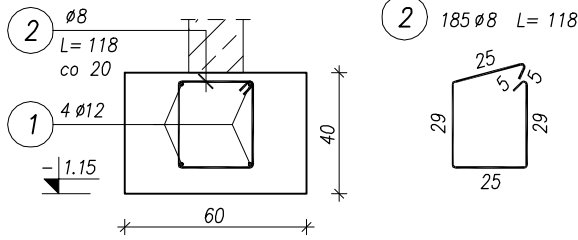
4.1 ława fundamentowa skala 1:25
