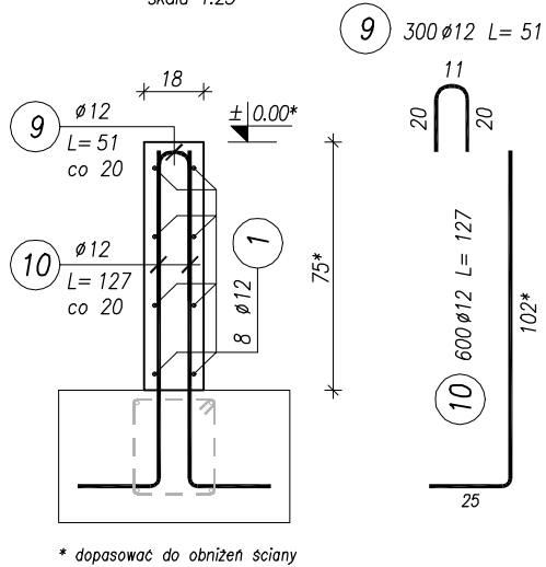
SF-1 ściana fundamentowa skala 1:25
