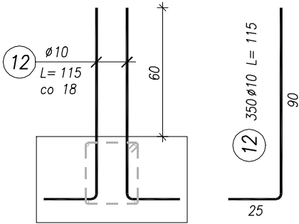
K-2 wykotwienie ścian skala 1:25
