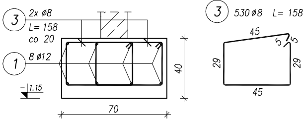
4.2 ława fundamentowa skala 1:25
